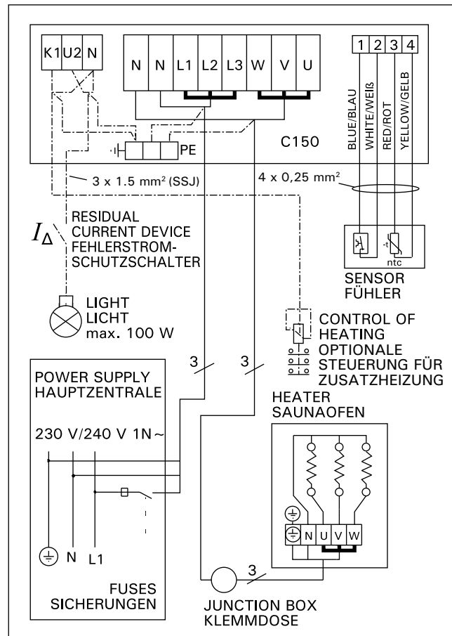
Figure 10b. 1-phase electrical connections of control unit C150 and PI-E-heater Abbildung 10b. 1-phasiger Elektroanschlüsse des Steuergerät C150 und des Saunaofens PI-E
