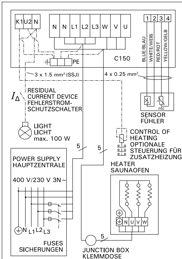
Figure 10a. 3-phase electrical connections of control unit C150 and PI-E-heater Abbildung 10a. 3-phasiger Elektroanschlüsse des Steuergerät C150 und des Saunaofens PI-E
